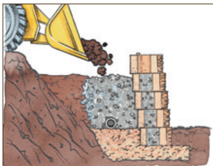
Diagram 7—Backfill
